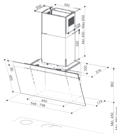
Minimální vzdálenost od varné desky 450 / 650 mm (plyn).
