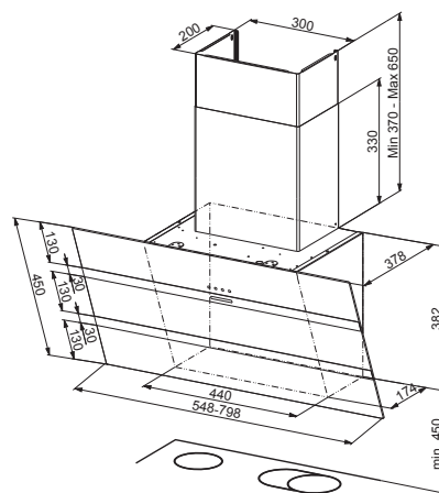
Minimální vzdálenost od varné desky 450 mm.
